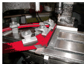
... an unserer Fräsmaschine
