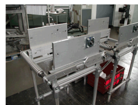
Vormontage in der Werkstatt
